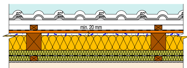
TŘÍPLAŠŤOVÁ STŘEŠ S VĚTRÁNÍM NAD I POD BEDNĚNÍM
