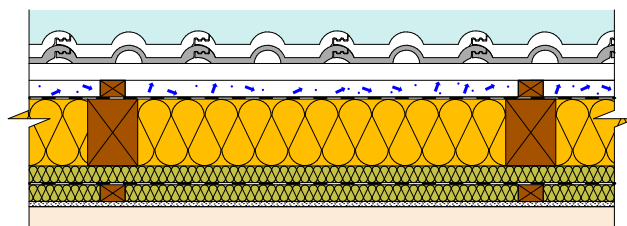
DVOUPLAŠŤOVÁ VĚTRANÁ STŘEŠ S VĚTRÁNÍM NAD FÓLIÍ
