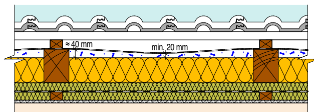
TŘÍPLAŠŤOVÁ STŘEŠ S VĚTRÁNÍM NAD I POD FÓLIÍ
